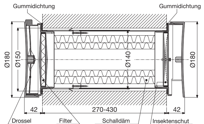
Außengitter, Typ 1
