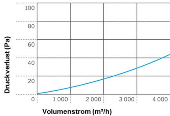
Anfangsdruckverlust Für Filtergröße 592 x 592 x 360 mm
